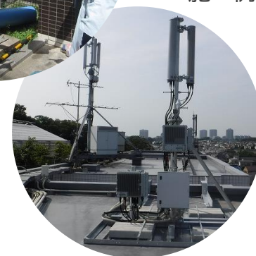
アンテナ工事 施工例
